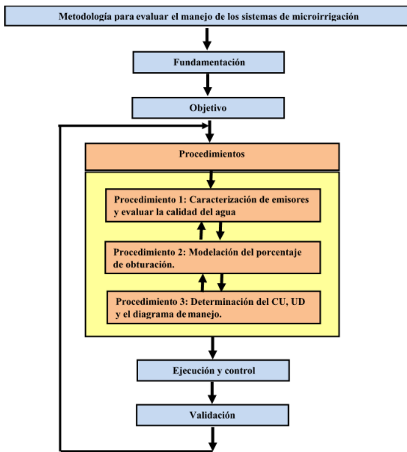
FIGURA 2. Esquema de la metodología propuesta para evaluar el manejo de los sistemas de microirrigación en Ciego de Ávila.
