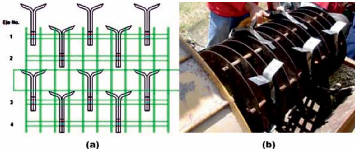
FIGURA 3. Distribución de cuchillas; (a) vista esquemática eje 1 a 4; (b) construidas y acopladas.
