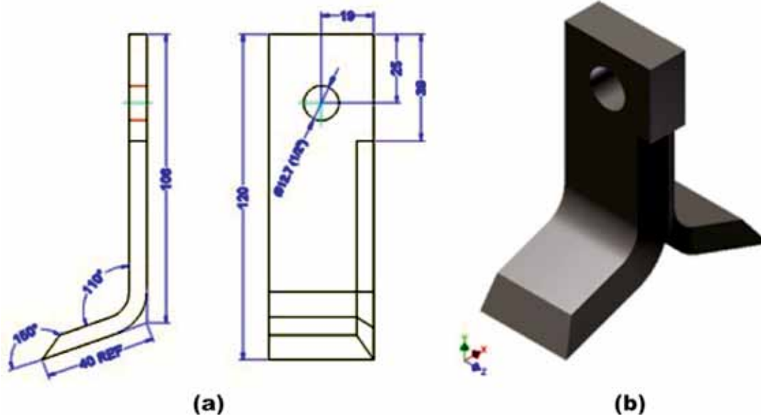
FIGURA 2. Cuchilla; (a) ½”Y” dimensiones; (b)”Y” modelado 3D en Autodesk Inventor 2010.
