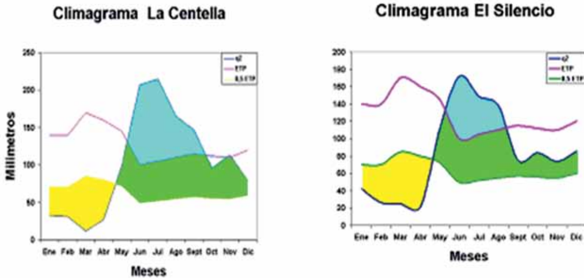
FIGURA 9. Climagramas de los pluviómetros comprendidos. Ejemplo en el polígono 3.
