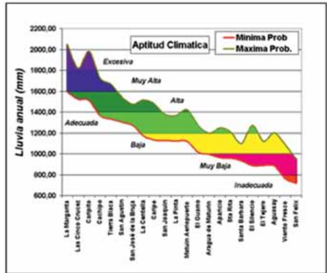
FIGURA 7. Lluvia total anual, máxima y mínima probable, para todos los pluviómetros analizados.
