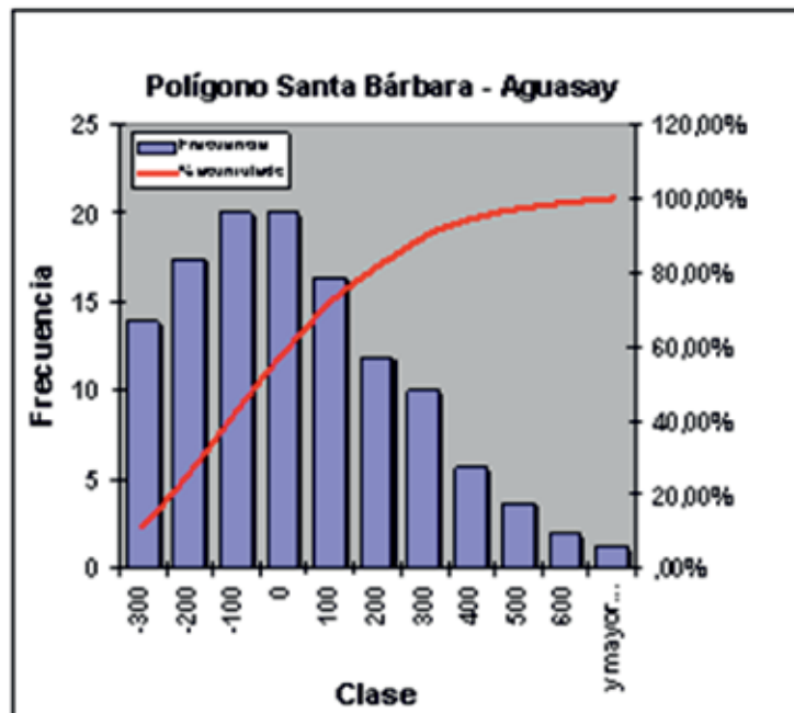
FIGURA 8. Probabilidad de ocurrencia de años con necesidades de suministro adicional de agua para el cultivo de la caña de azúcar. Ejemplo Polígono 1.
