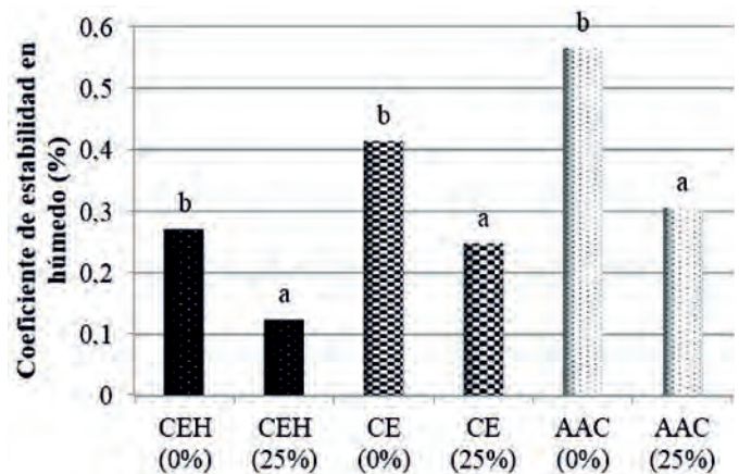
FIGURA 4. Análisis de estabilidad estructural de los agregados en el tamizado en húmedo.
