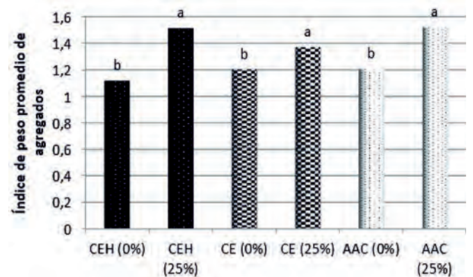
FIGURA 5. Índice de peso promedio de agregados ponderado por diámetro de los suelos en estudio.
