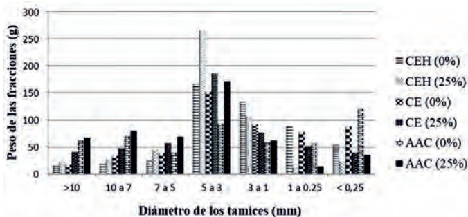
FIGURA 1. Distribución de agregados en el tamizado en seco para los suelos en estudio.
