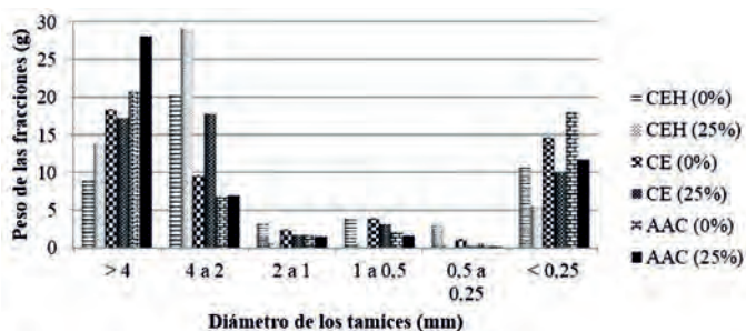
FIGURA 2. Distribución de agregados en el tamizado húmedo para los suelos en estudio.
