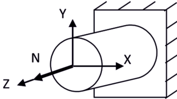
FIGURA 5. Sentido de la fuerza de tracción N.
