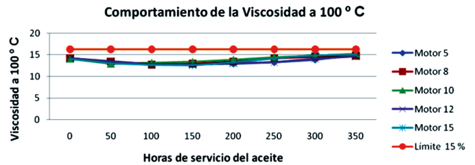
FIGURA 4. Comportamiento de la viscosidad a 100 °C.
