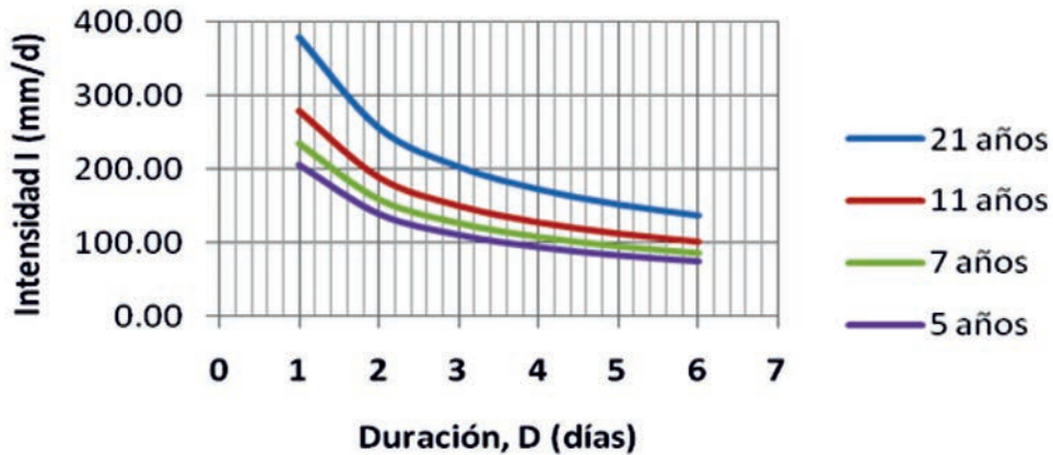
FIGURA 5. Curva de IFD de las inundaciones para T = 12, 11, 7 y 5 años.
