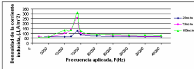
FIGURA 5. Densidad máxima de la corriente inducida en el enrollado receptor en función de la frecuencia de la excitación del enrollado emisor, para una distancia entre enrollados de 50 cm y diferentes valores de la conductividad eléctrica del suelo.
