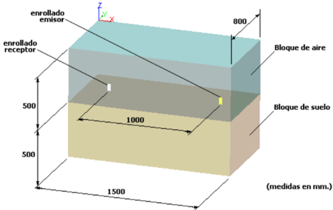
FIGURA 1. Modelación digitalizada del sistema suelo-aire-electrodos.
