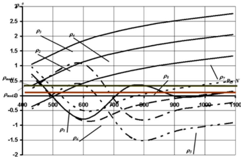
FIGURA 7. Gráfica de la variación del valor del ángulo de giro de la barra principal del arado FDN, \rho , en función del valor de la fuerza de resistencia al tiro (horizontal) R_x , y su relación con los valores de la fuerza R_z (Figuras 3 y 4) para lograr su estabilidad estática, con \beta = 20^\circ (Figuras 1 y 2 y Tablas 1 y 2) y donde: \rho_1 - a = 0,15 m, Z_1 = (1/4).a , \alpha = 25^\circ ; \rho_2 - a = 0,15 m, Z_1 = (1/3).a , \alpha = 25^\circ ; \rho_3 - a = 0,15 m, Z_1 = (1/4).a , \alpha = 35^\circ ; \rho_4 - a = 0,15 m, Z_1 = (1/3).a , \alpha = 35^\circ ; \rho_5 - a = 0,25 m, Z_1 = (1/4).a , \alpha = 25^\circ ; \rho_6 - a = 0,25 m, Z_1 = (1/3).a , \alpha = 25^\circ ; \rho_7 - a = 0,25 m, Z_1 = (1/4).a , \alpha = 35^\circ ; \rho_8 - a = 0,25 m, Z_1 = (1/3).a , \alpha = 35^\circ . Los valores medios del ángulo de giro de la barra principal del arado FDN para p = 0,95 son: \rho_{med1} = 0,5764 \pm 0,472^\circ , para Z_1 = (1/4).a y \rho_{med2} = 0,3376 \pm 0,4758^\circ , para Z_1 = (1/3).a . Nota: c = 40 mm.
