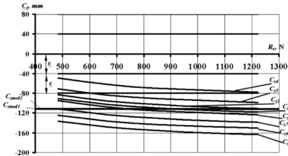
FIGURA 8. Gráfica de la variación del de la distancia de regulación vertical C_2 , mm del punto de tiro del arado FDN con la barra de tiro A, en función del valor de la fuerza de resistencia al tiro (horizontal) R_x , y su relación con los valores de la fuerza R_z (Figuras 3 y 4) para lograr su estabilidad estática, con \beta = 18^\circ (Figuras 1 y 2 y Tablas 1 y 2) y donde: C_{21} - a = 0,15 m, Z_1 = (1/4).a , \alpha = 25^\circ ; C_{22} - a = 0,15 m, Z_1 = (1/3).a , \alpha = 25^\circ ; C_{23} - a = 0,15 m, Z_1 = (1/4).a , \alpha = 35^\circ ; C_{24} - a = 0,15 m, Z_1 = (1/3).a , \alpha = 35^\circ ; C_{25} - a = 0,25 m, Z_1 = (1/4).a , \alpha = 25^\circ ; C_{26} - a = 0,25 m, Z_1 = (1/3).a , \alpha = 25^\circ ; C_{27} - a = 0,25 m, Z_1 = (1/4).a , \alpha = 35^\circ ; C_{28} - a = 0,25 m, Z_1 = (1/3).a , \alpha = 35^\circ . Los valores medios de la distancia de regulación vertical del punto de tiro del arado FDN con la barra de tiro A para p = 0,95 son: C_{2med1} = -112,5729 \pm 13,2327 , mm para Z_1 = (1/4).a y C_{2med2} = -111,5282 \pm 13,2486 , mm para Z_1 = (1/3).a . Nota: c = 40 mm.
