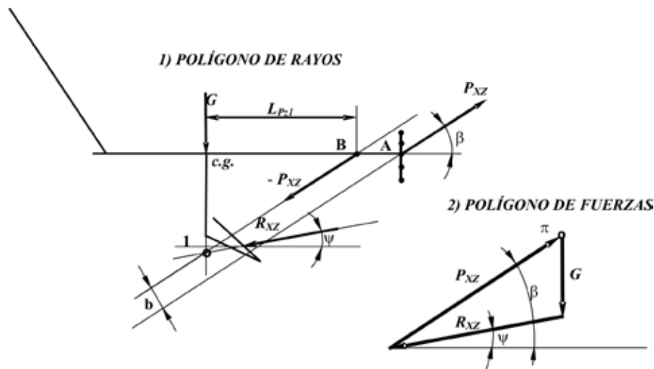
FIGURA 1. Esquema de los Polígonos de 1) Fuerza y 2) de Rayos que estabilizan estáticamente a un arado de tiro animal.
