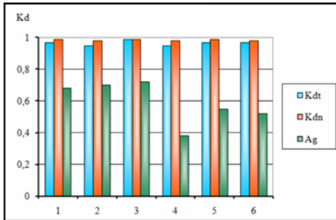
FIGURA 2. Comportamiento de los coeficientes de disponibilidad técnica K_{dt} , K_{dn} y de la disponibilidad genérica durante el período desde junio 2009-enero 2010.
