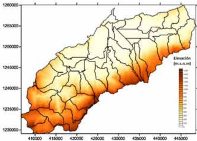
FIGURA 3. Delimitación automática de la cuenca y subcuencas del río Coro hasta el punto de cierre.
