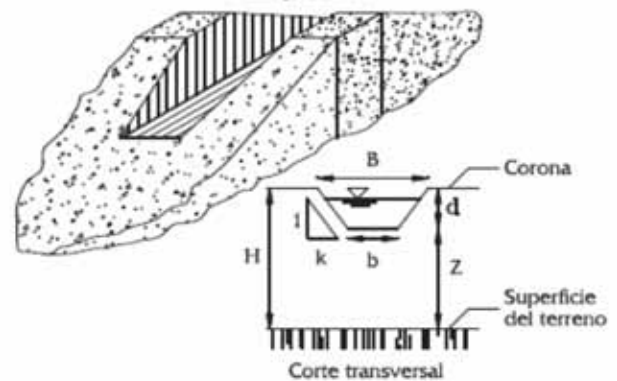
FIGURA 5. Forma y dimensiones de la brecha.
