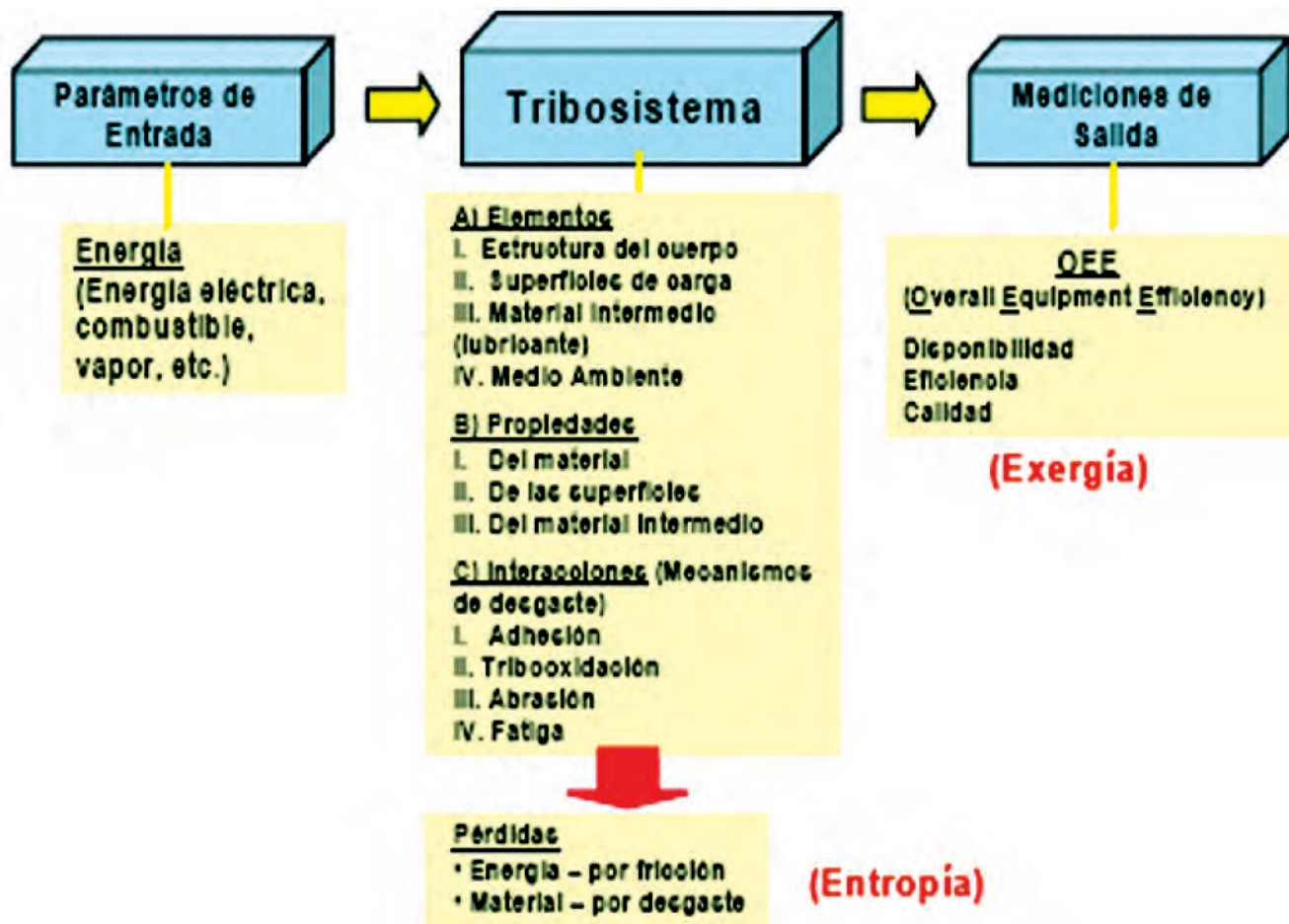
FIGURA 4. Análisis tribotermodinámico de un tribosistema.
