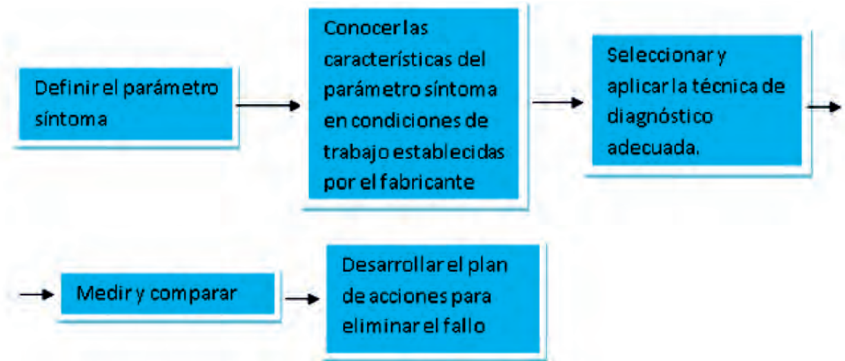
FIGURA 5. Secuencia de pasos para determinar fallos.
