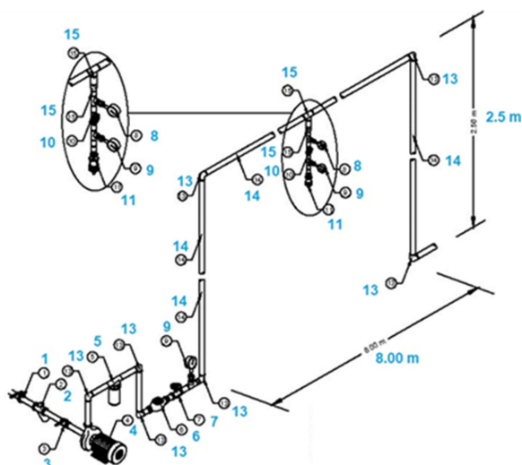
FIGURA 7. Pódico y componentes de la instalación hidráulica para la evaluación de boquillas difusoras MPCE a diferentes alturas.
